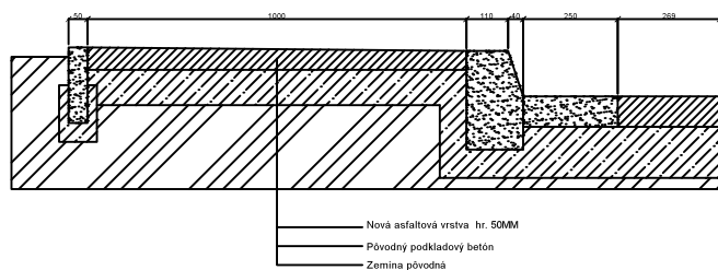
V3 Verzia 3 - fasáda - cestný obrubník
