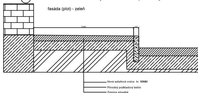
V6 Verzia 6 - fasáda - záhonový obrubník bez prídlažby
