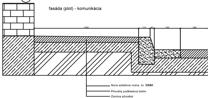
V3 Verzia 3 - fasáda - cestný obrubník
