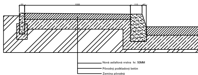
V6 Verzia 6 - fasáda - záhonový obrubník bez prídlažby
