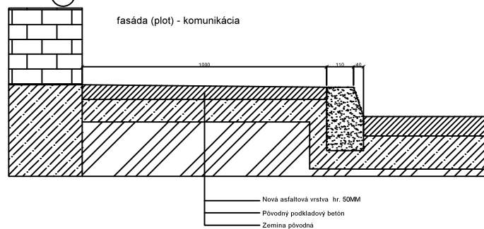
V4 Verzia 4 - fasáda - cestný obrubník bez prídlažby
